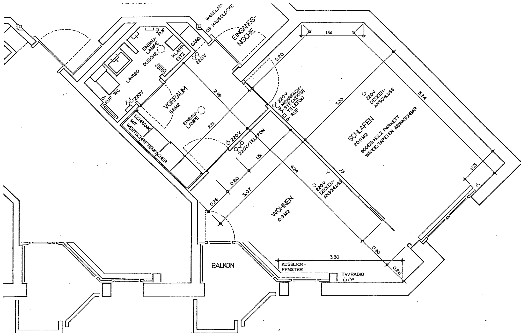
2-ER PENSIONÄRZIMMER MIT EINBAUMOBILIAR, MASSEN UND ELEKTRONSTALLATIONEN
