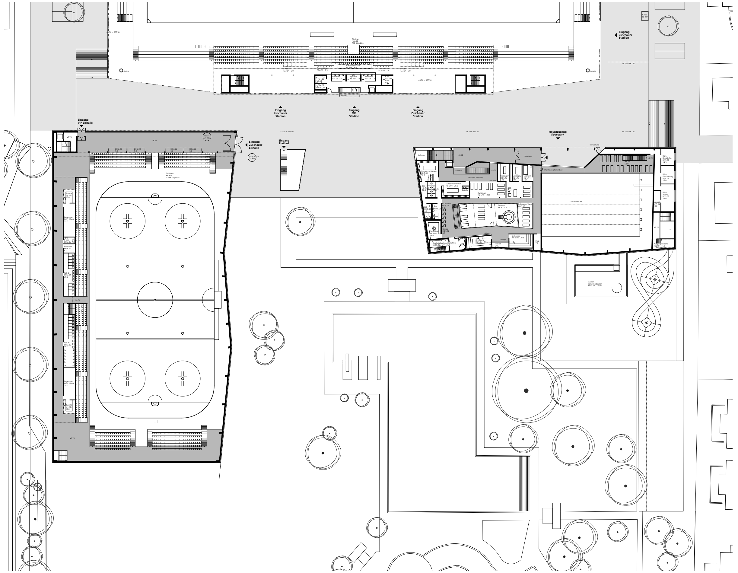
Grundriss Ebene +1 / Eishalle - Hallenbad - Freibad
