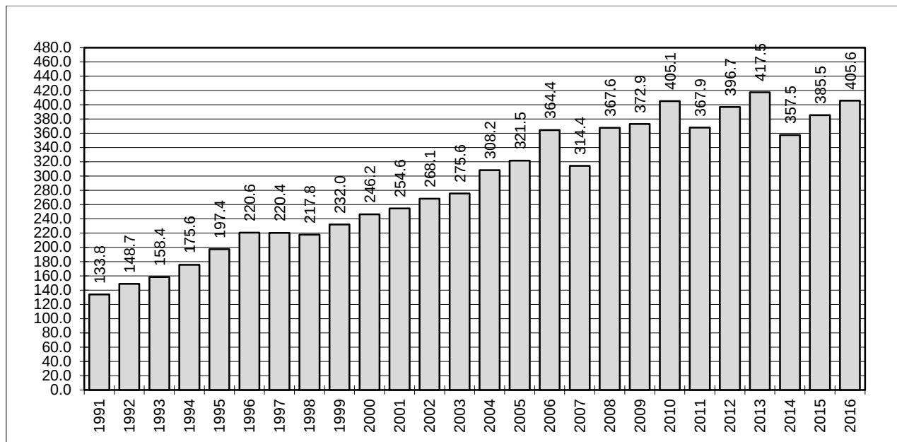
Gasabsatz 1991-2016 in Mio. kWh (bis 2009 hydrologisches Jahr / ab 2010 Kalenderjahr)
